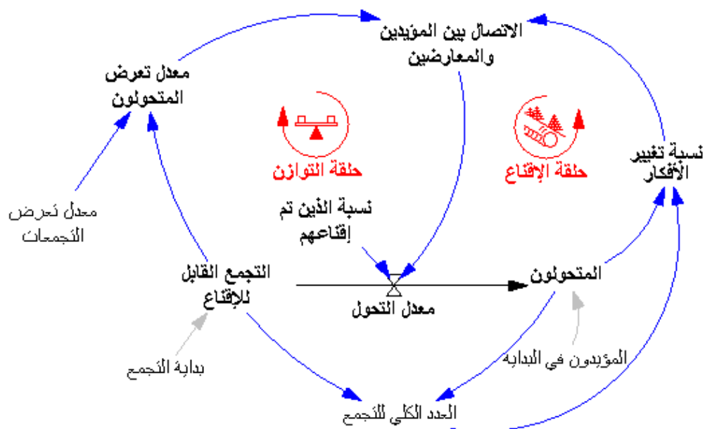
شكل (4): التمثيل الديناميكي لنقل الأفكار وعدوى الشائعات
