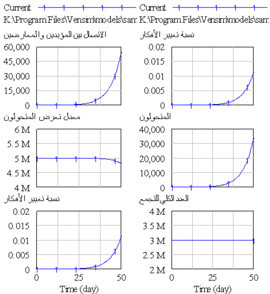
شكل (6): النتائج العددية لنموذج انتقال الشائعات في تجمع عدده ثابت
