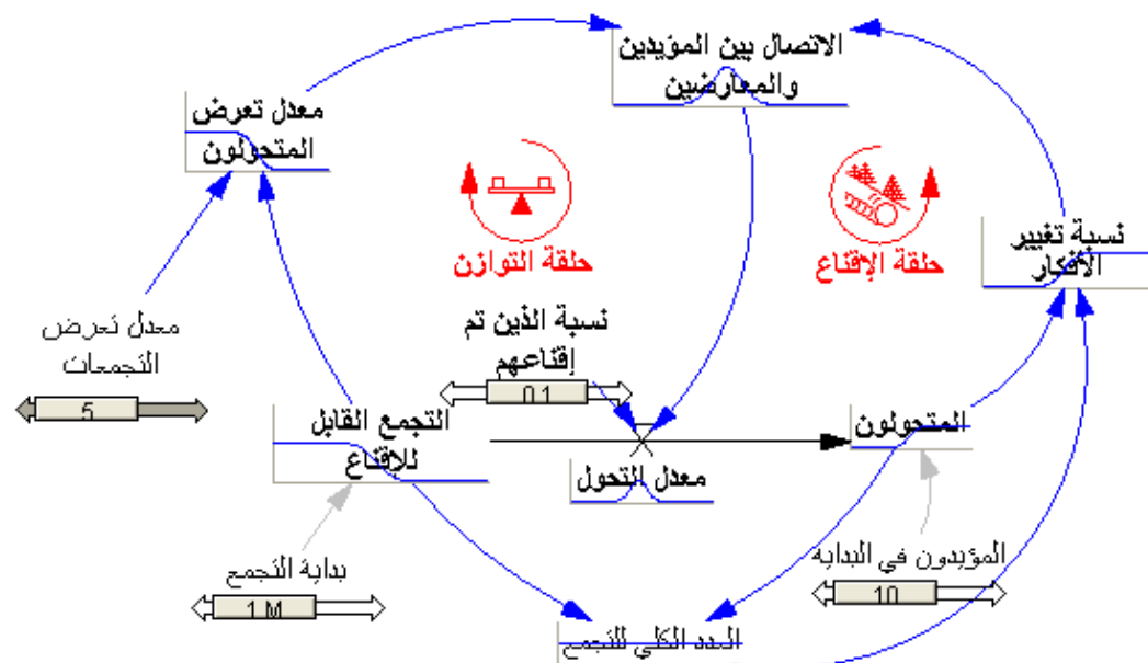
شكل (5): محاكاة النموذج العددي لانتقال الدعوة للإضراب
